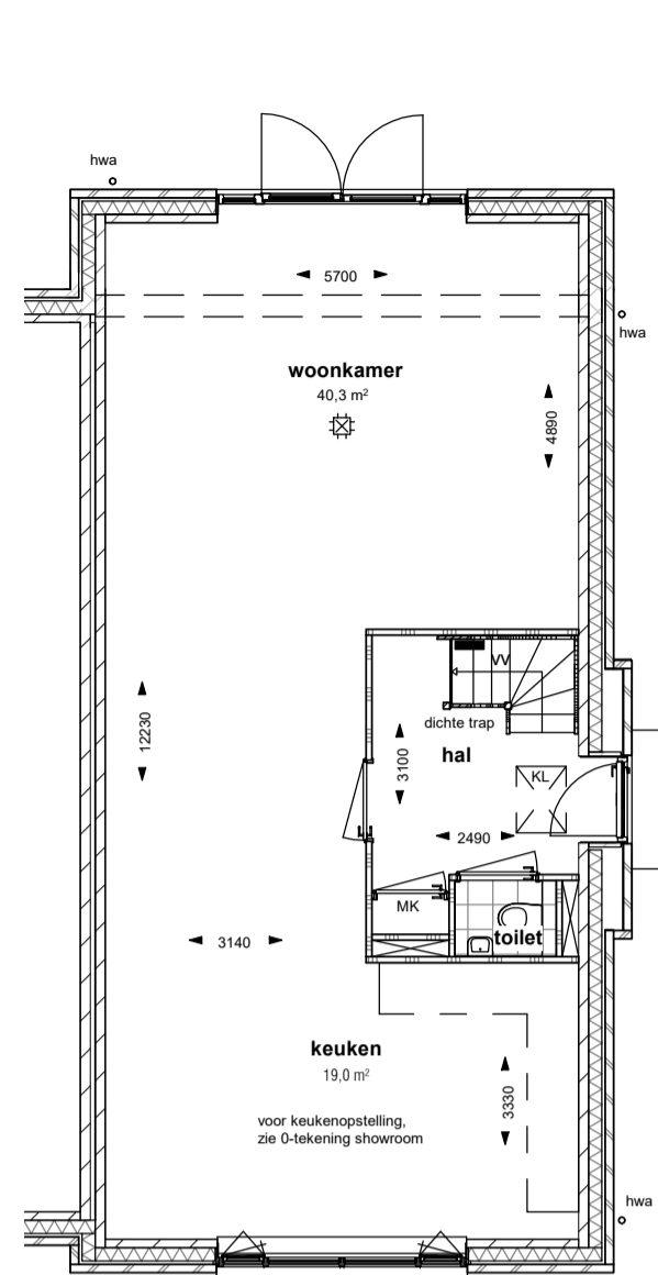
Optie uitbouw 1,2 meter SCHAAL: 1 : 100
