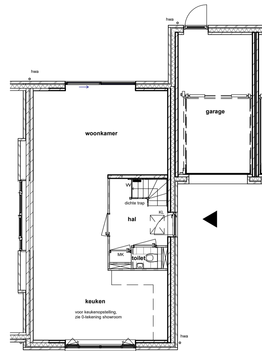
Optie schuifpui begane grond SCHAAL: 1 : 100
