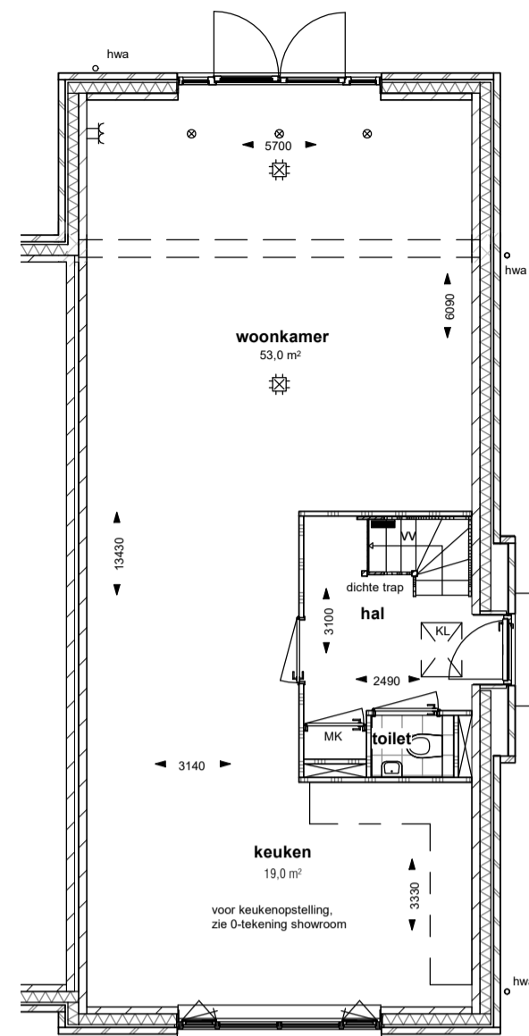
Optie uitbouw 2,4 meter SCHAAL: 1 : 100
