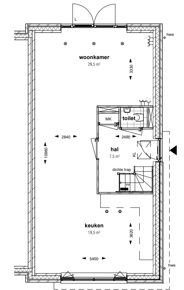
Optie tuingericht wonen begane grond SCHAAL: 1 : 100
