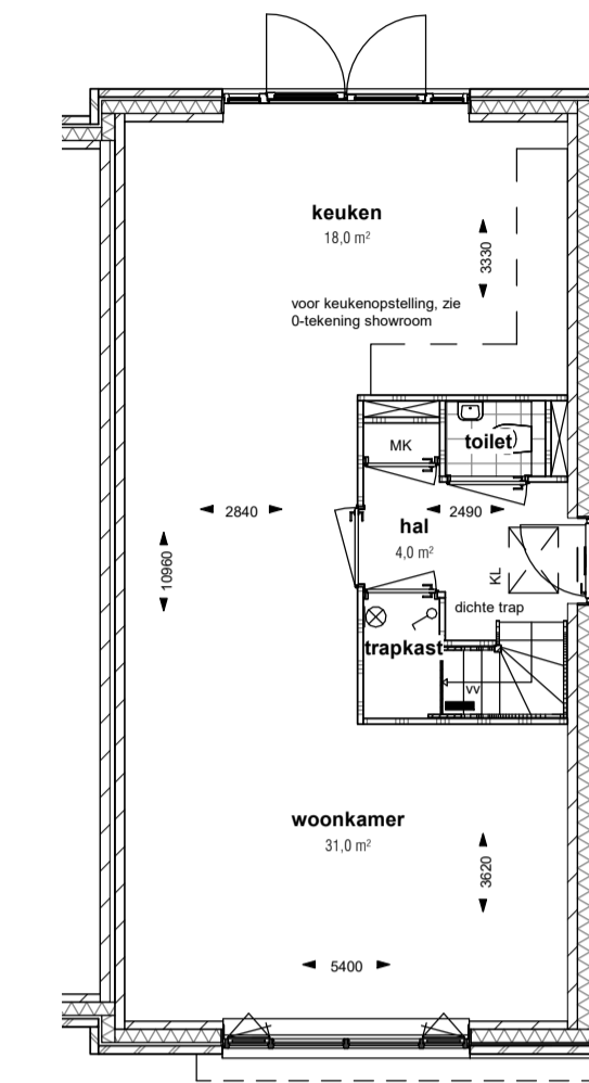
Optie trapkast SCHAAL: 1 : 100
