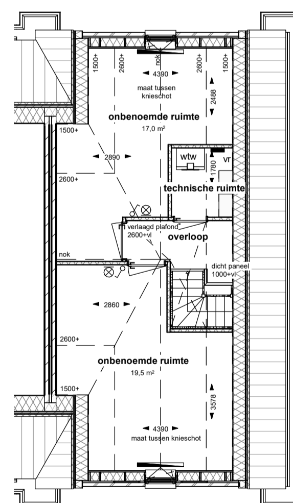
Optie indeling zolder 2 kamers SCHAAL: 1 : 100
