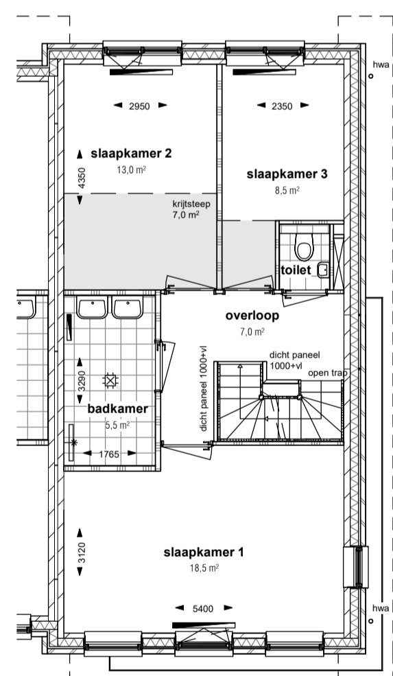
Optie vergroten badkamer 500mm SCHAAL: 1 : 100
