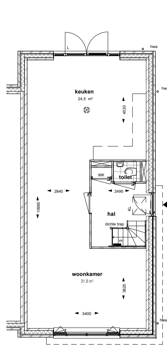
Optie uitbouw 1,2 meter begane grond SCHAAL: 1 : 100
