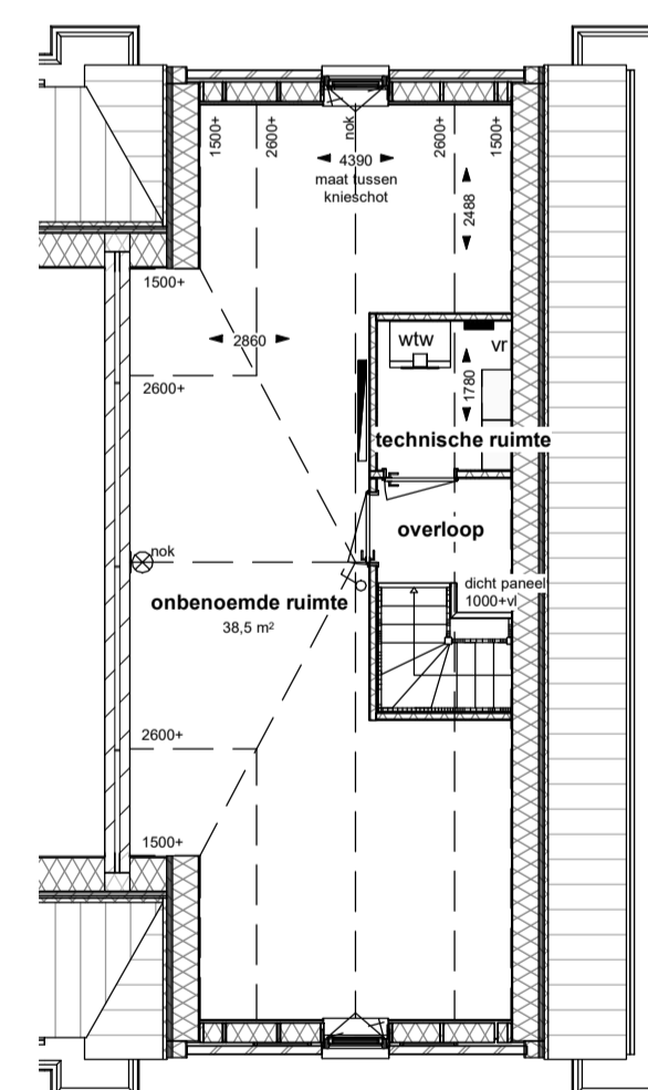
Optie indeling zolder 2e verdieping SCHAAL: 1 : 100
