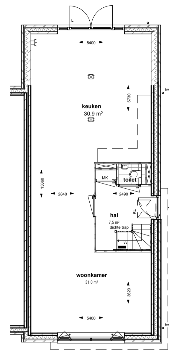
Optie uitbouw 2,4 meter begane grond SCHAAL: 1 : 100
