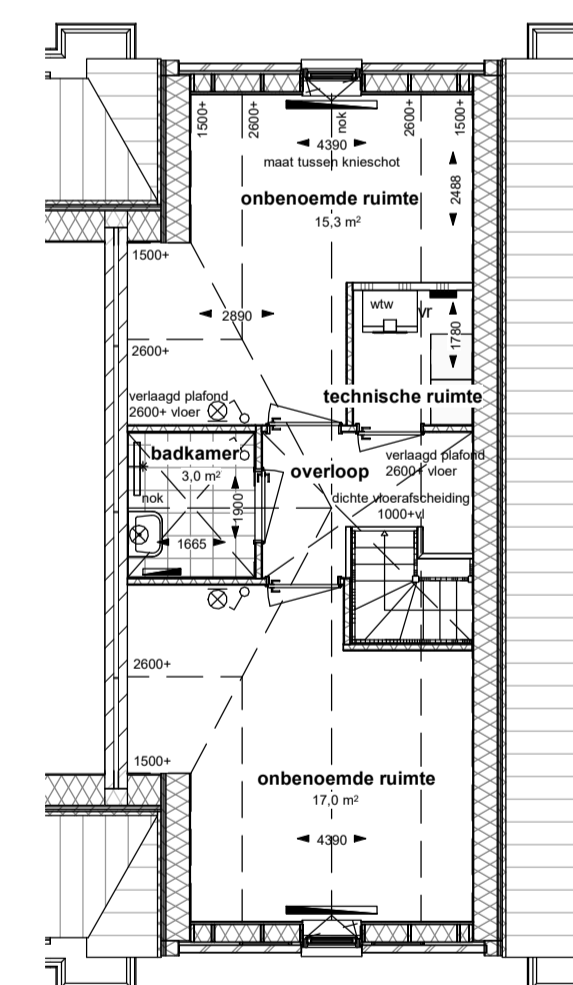
Optie badkamer op zolder SCHAAL: 1 : 100
