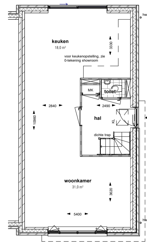
Optie schuifpui SCHAAL: 1 : 100
