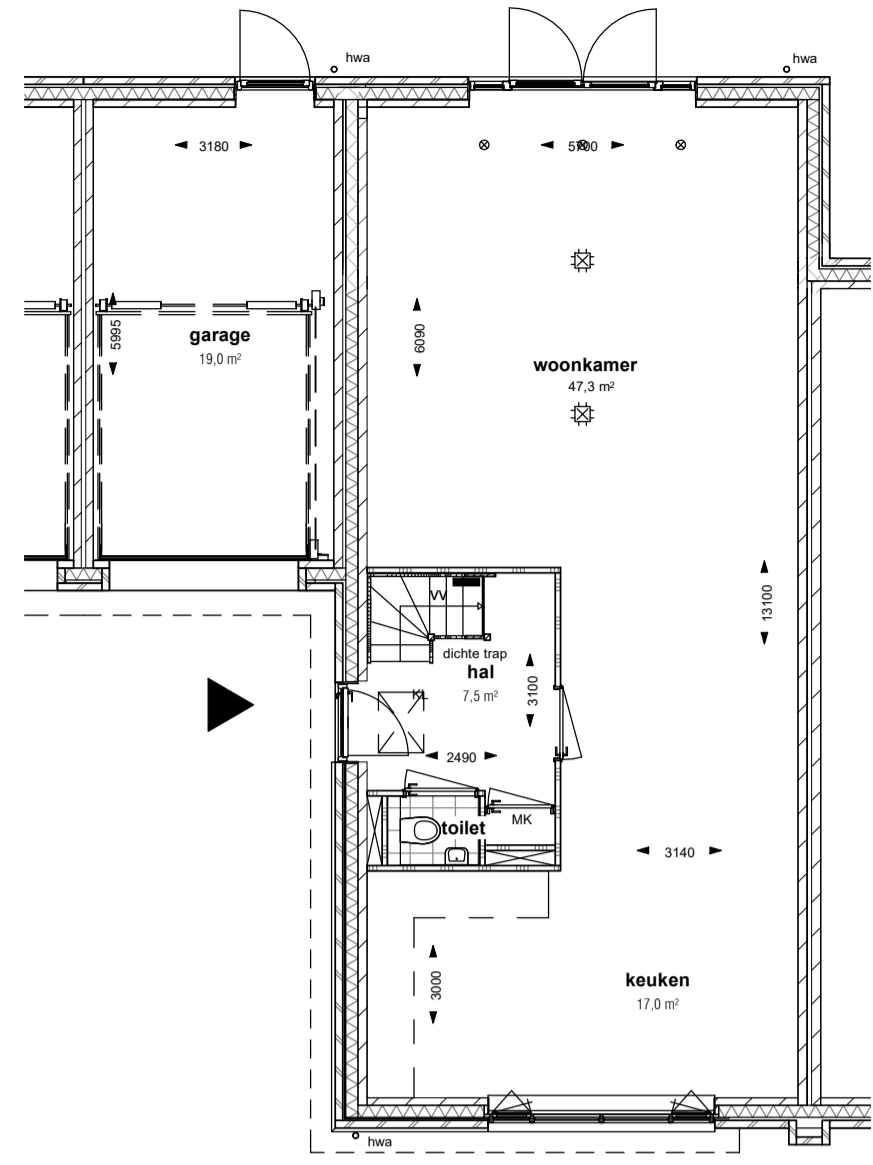
Optie uitbouw 2,4 meter begane grond SCHAAL: 1 : 100
