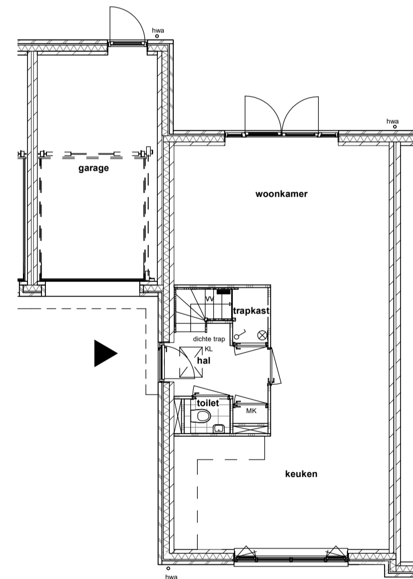
Optie trapkast SCHAAL: 1 : 100
