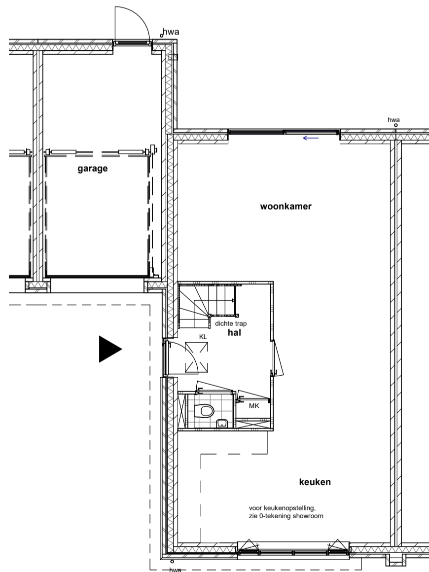
Optie schuifpui SCHAAL: 1 : 100
