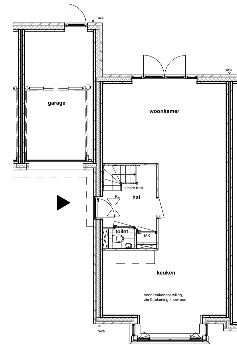
Optie erker SCHAAL: 1 : 100
