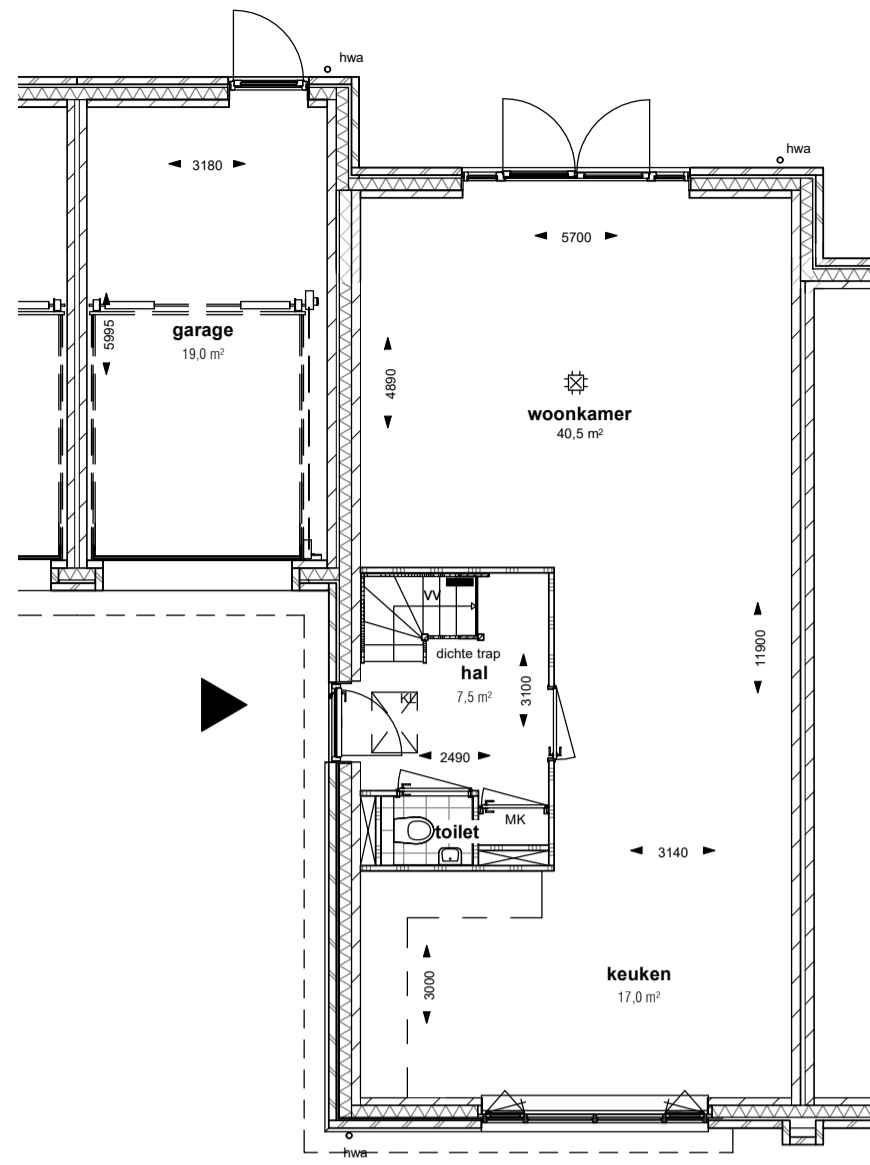
Optie uitbouw 1,2 meter begane grond SCHAAL: 1 : 100
