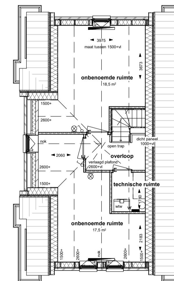
Optie indeling zolder in 2 ruimtes SCHAAL: 1 : 100
