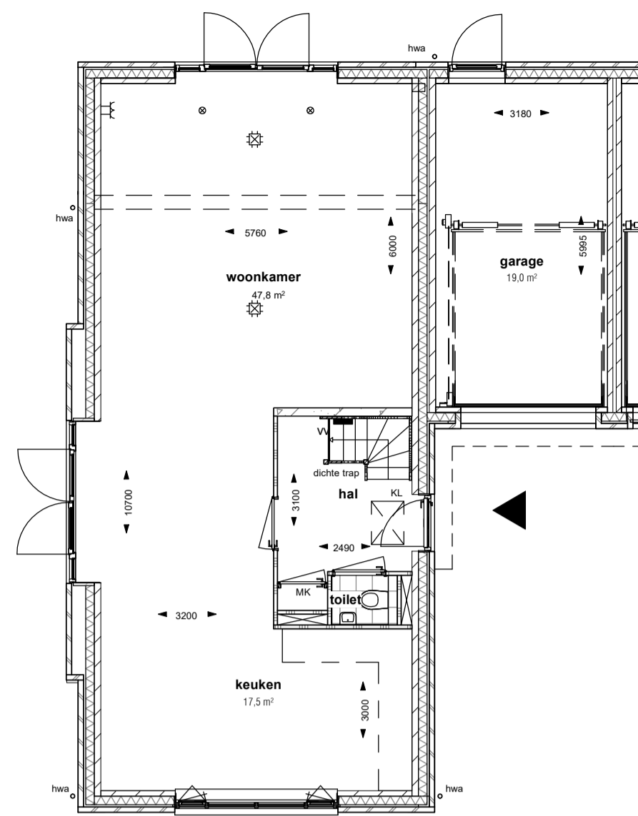
Optie uitbouw 2,4 meter begane grond SCHAAL: 1 : 100
