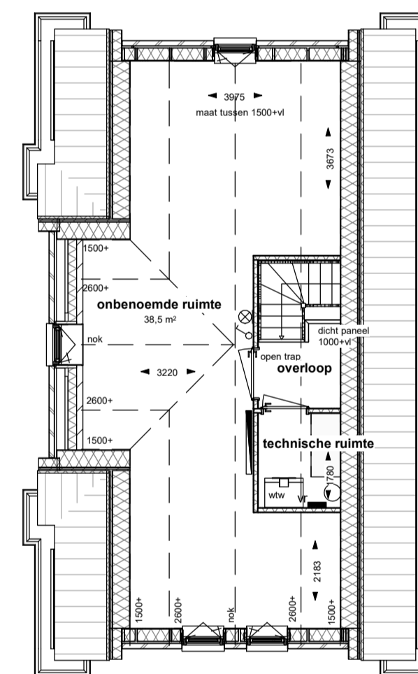
Optie indeling zolder SCHAAL: 1 : 100
