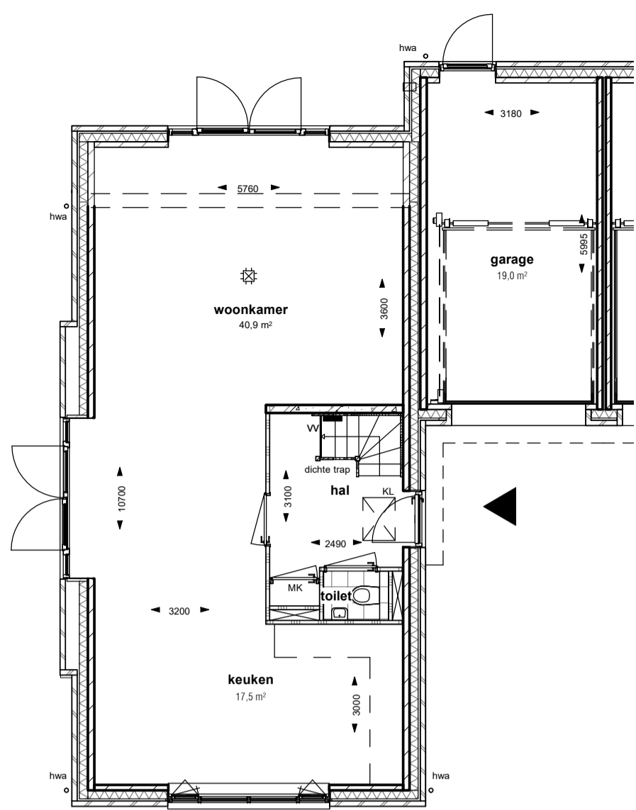
Optie uitbouw 1,2 meter begane grond SCHAAL: 1 : 100
