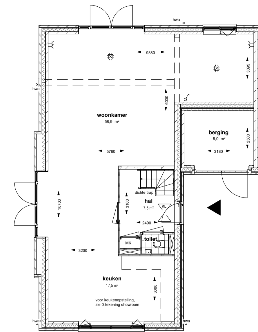
Optie uitbouw splitsing garage SCHAAL: 1 : 100
