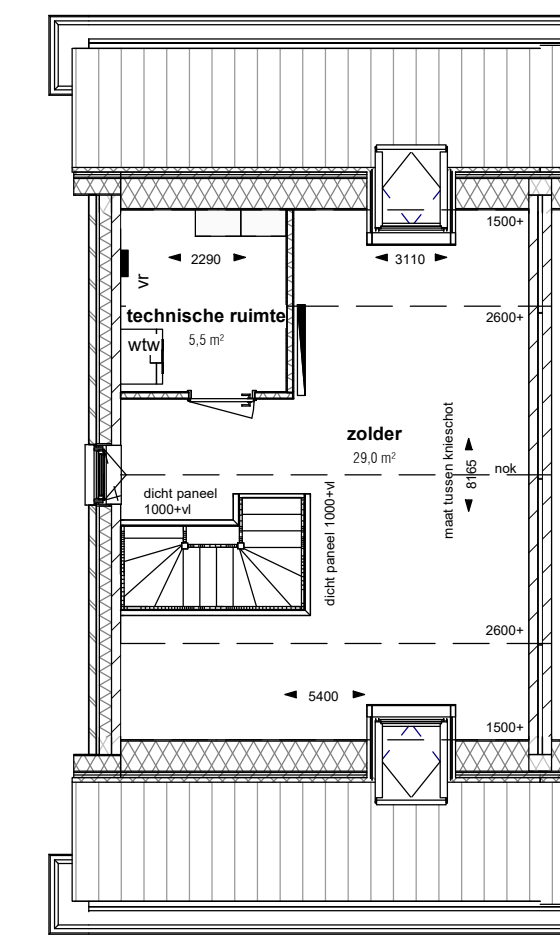
Optie dakraam 940x1400mm voor en/of achter SCHAAL: 1 : 100
