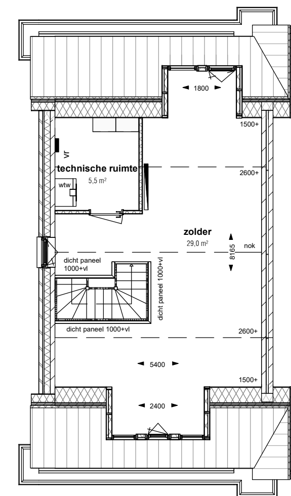
Optie dakkapel voor en/of achter SCHAAL: 1 : 100
