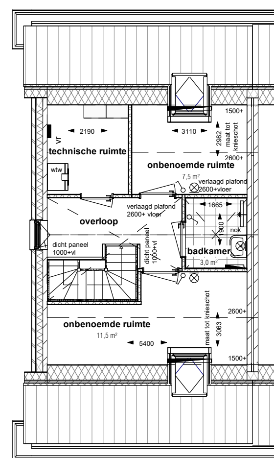
Optie badkamer op zolder SCHAAL: 1 : 100 incl 2 dakramen
