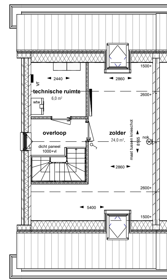
Optie indeling zolder incl. 2 dakramen SCHAAL: 1 : 100
