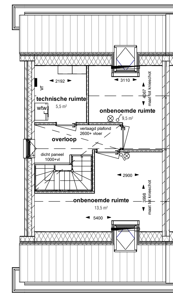
Optie indeling zolder in twee ruimtes SCHAAL: 1 : 100 incl 2 dakramen
