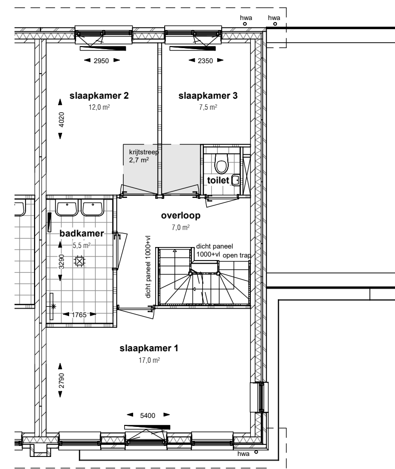
Optie vergroten badkamer 500mm richting slk 1 SCHAAL: 1 : 100
