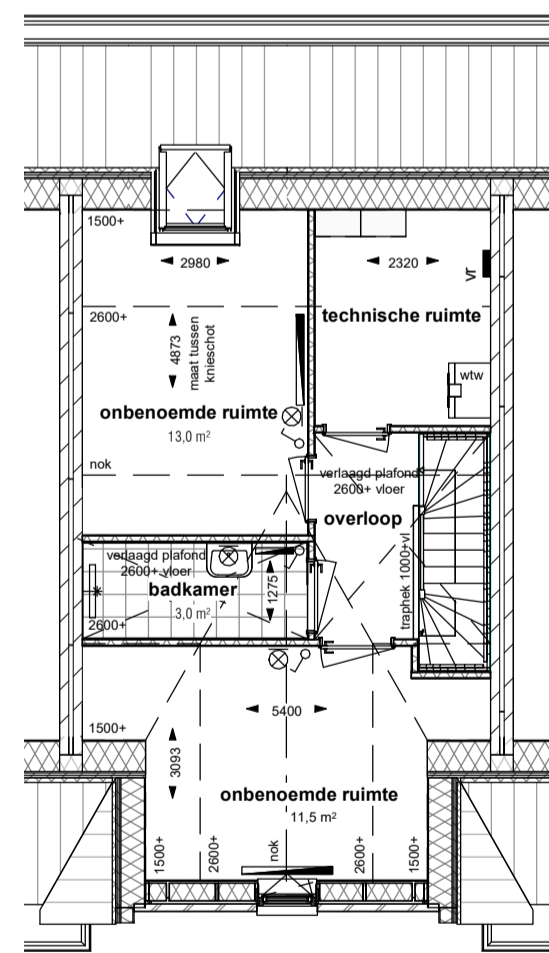
Optie badkamer op zolder SCHAAL: 1 : 100 incl 1 dakraam
