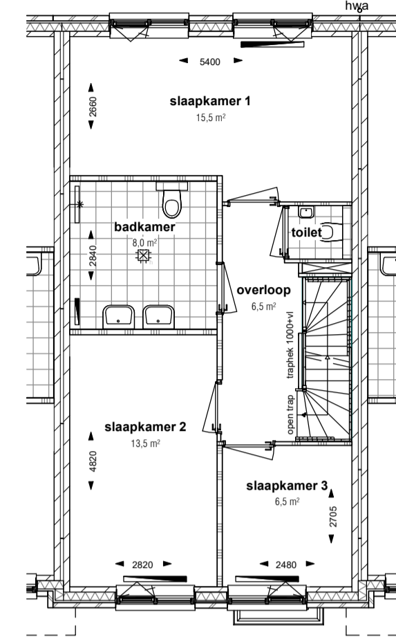
Optie vergroten badkamer 500mm SCHAAL: 1 : 100
