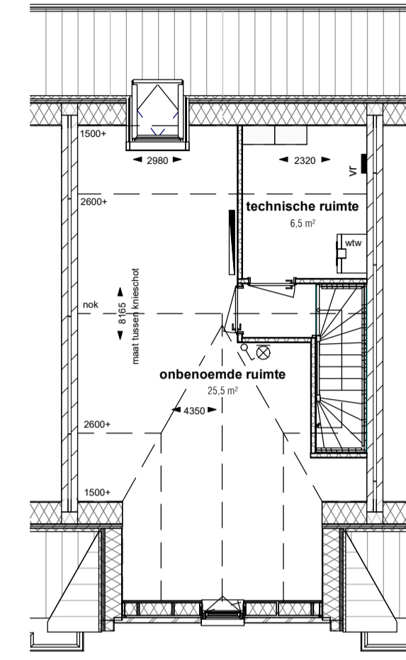
Optie indeling zolder incl. 1 dakraam SCHAAL: 1 : 100
