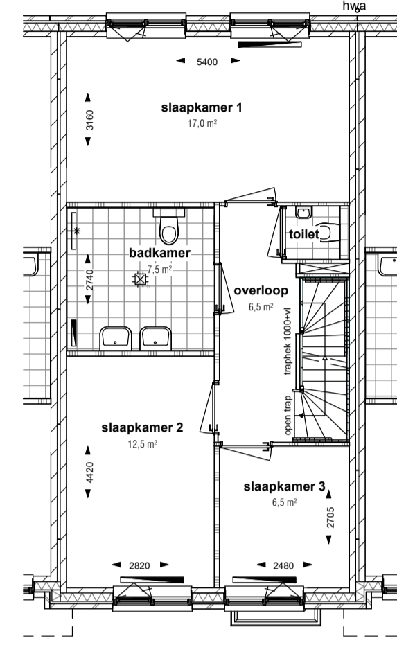
Optie vergroten badkamer 400mm SCHAAL: 1 : 100
