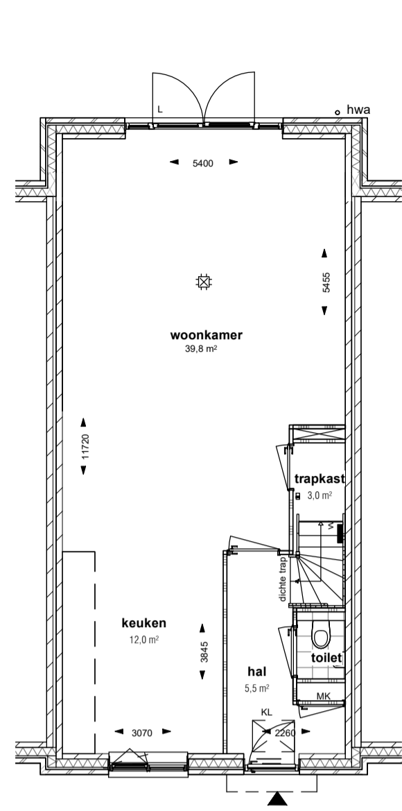
Optie uitbouw 1,2 meter begane grond SCHAAL: 1 : 100
