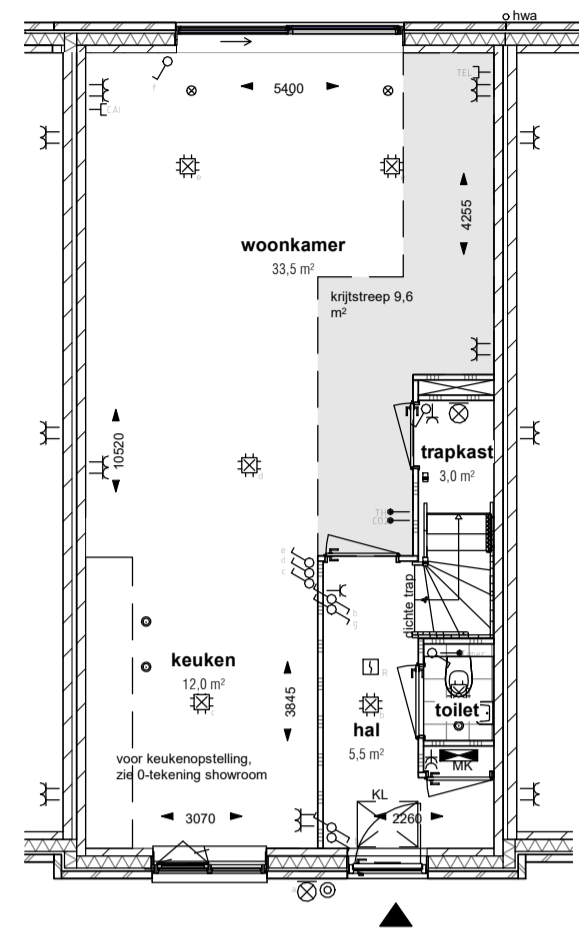
Optie schuifpui SCHAAL: 1 : 100
