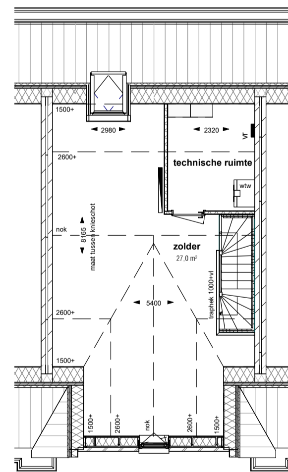
Optie dakraam 940x1400mm SCHAAL: 1 : 100
