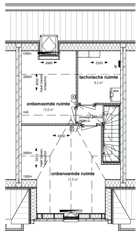
Optie indeling zolder SCHAAL: 1 : 100 incl 1 dakraam
