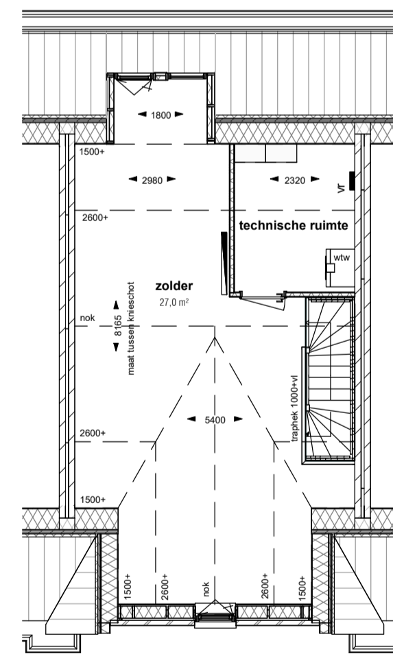
Optie dakkapel achter SCHAAL: 1 : 100
